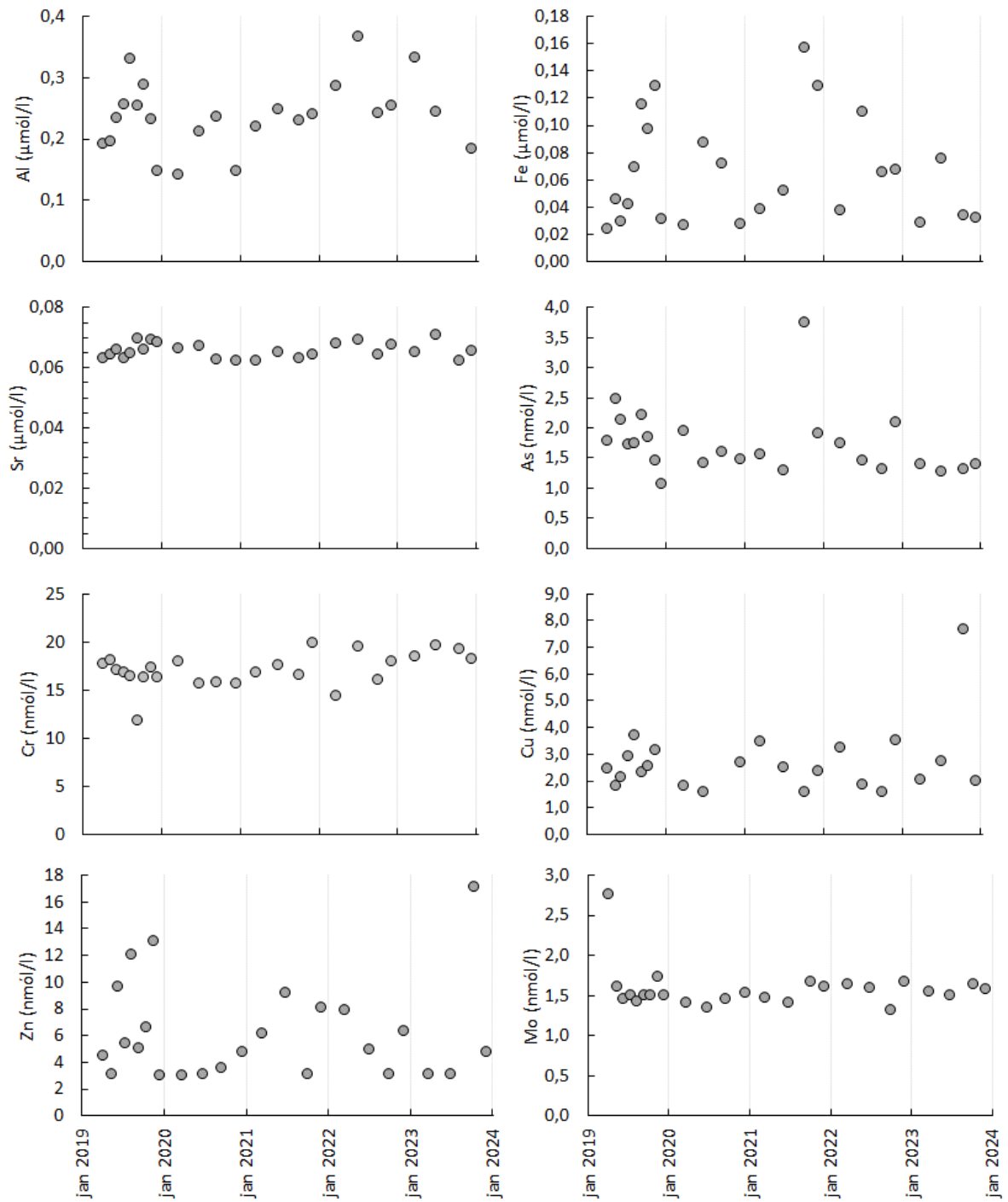
Mynd 5. Styrkur snefilefna í útfalli Þingvallavatns 2019-2023
