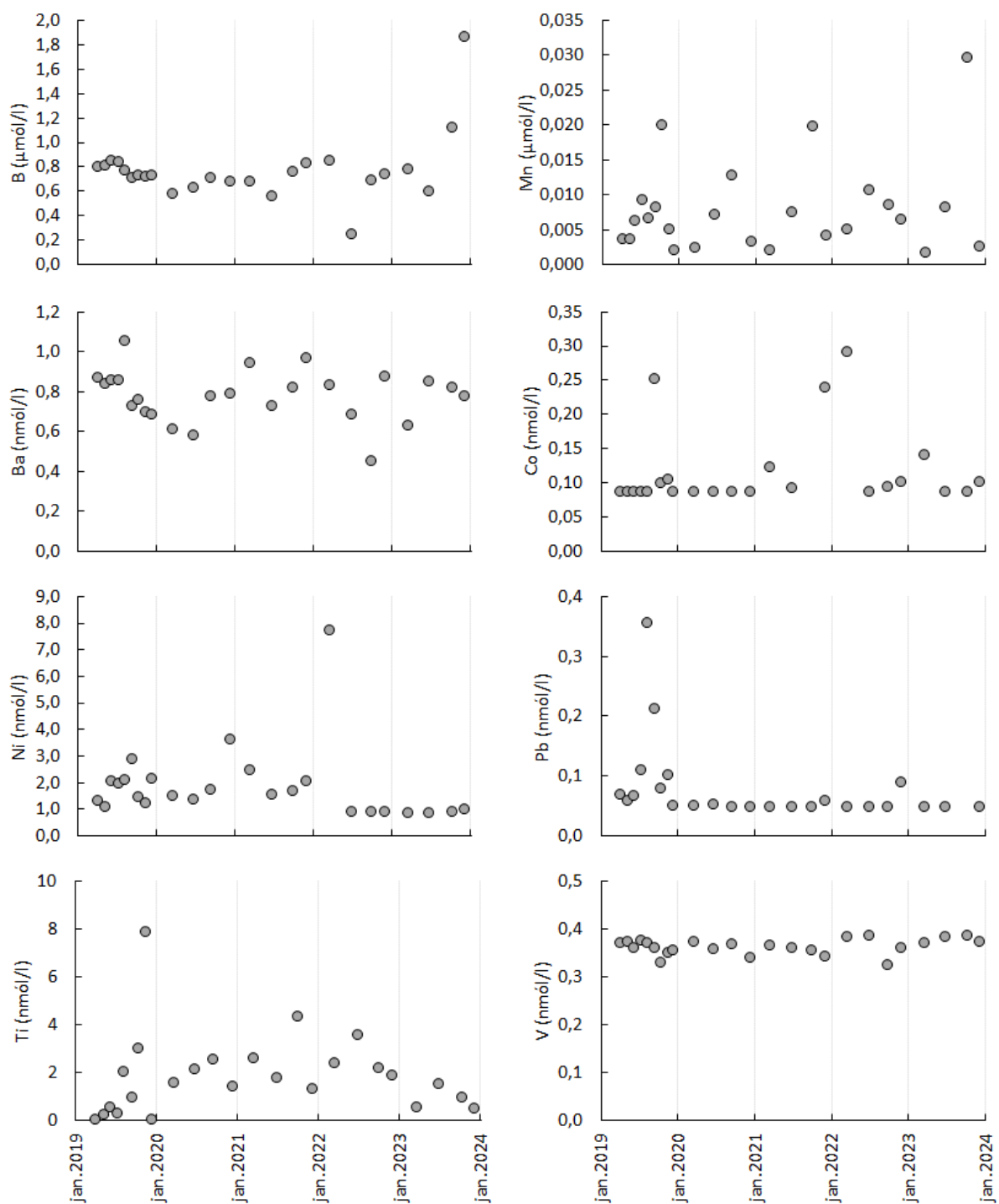
Mynd 6. Styrkur snefilefna í útfalli Þingvallavatns 2019-2023
